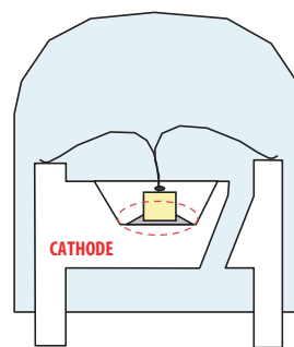
InGaN Device
