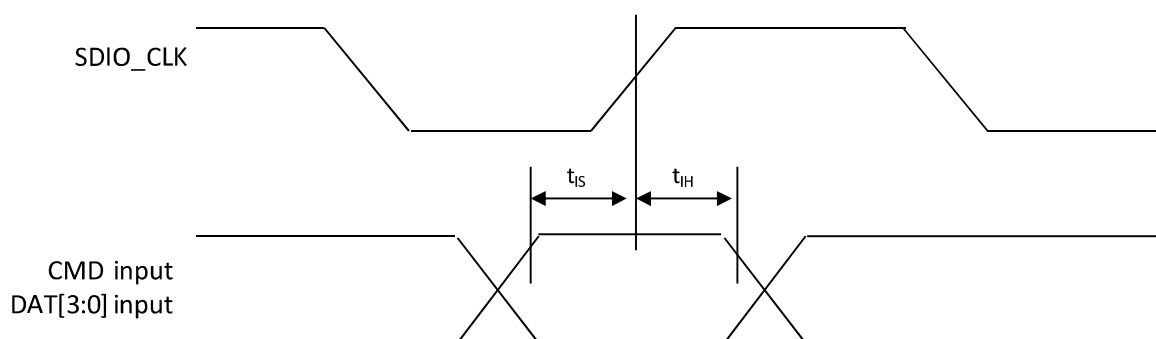
SDIO Bus Input Timing Parameters (SDR Modes)
