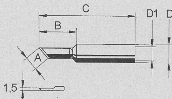
ERSA-832AD
