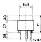
ST 1034 E 1-pole
