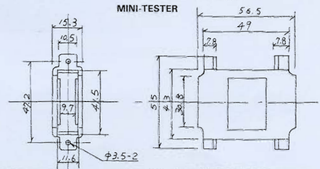
DD TYPE 50 PIN
