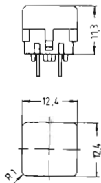
Abmessungen
